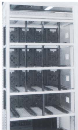
8E/4 和 8E/2 抽出式组件小室
