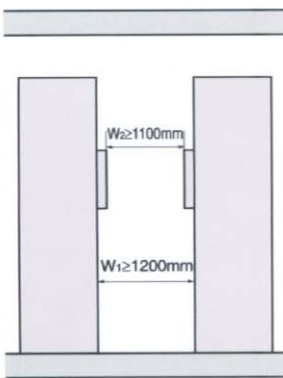
配电室安装尺寸及操作通道要求
