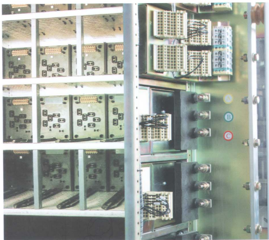
电缆和控制线在开关柜中的接线方式
