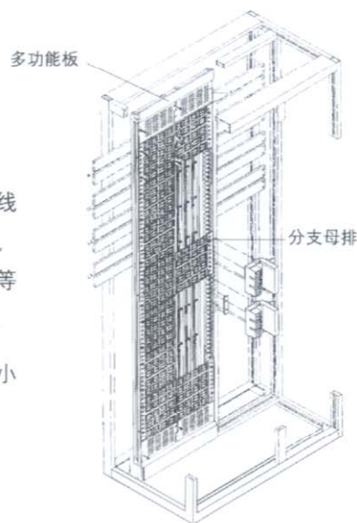
分支母排嵌入多功能分隔板中
