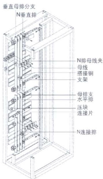
带母线、分支母线柜架
