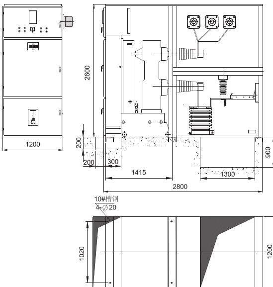
安装 40.5W-VAC、SF1、SF2 断路器
